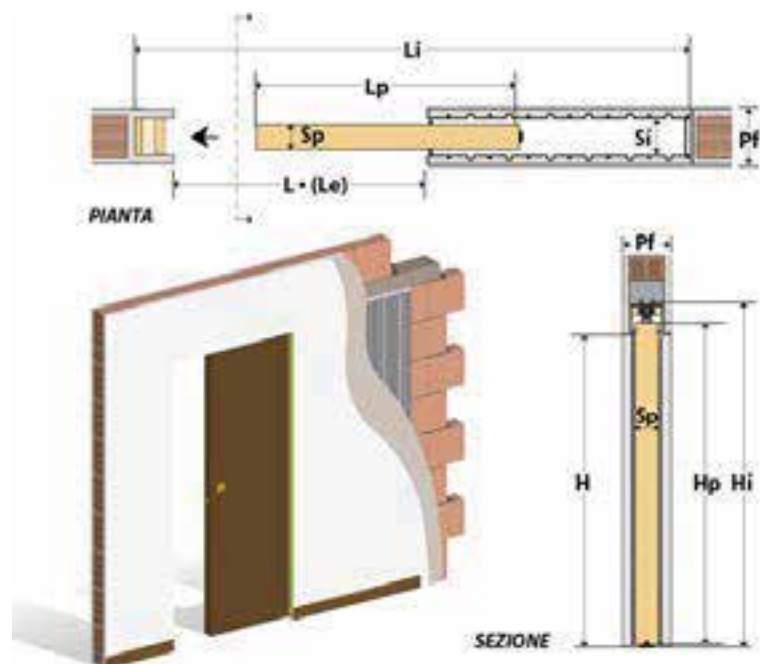
פרט לכיס בקו אפס ללא הלבשות
