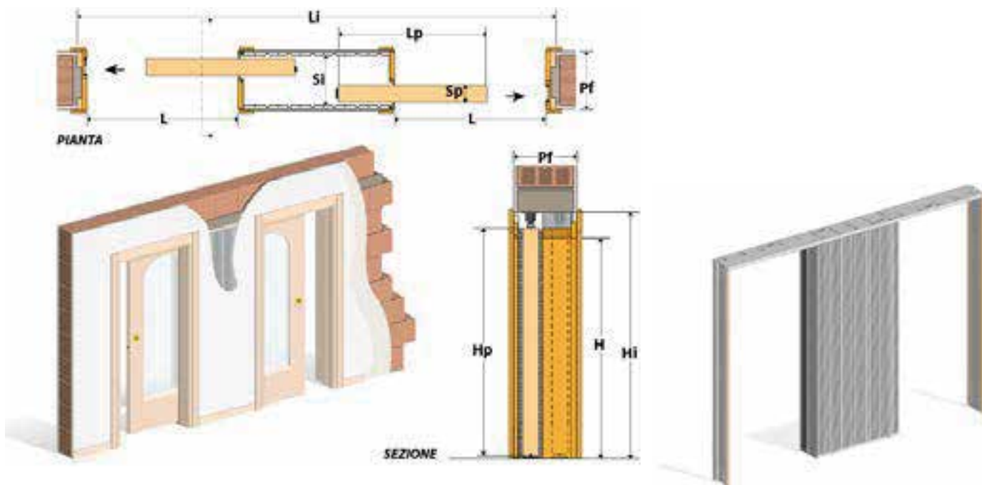
פרט לכיס בודד עם 2 דלתות נגררות נפתחות לצדדים מנוגדים
